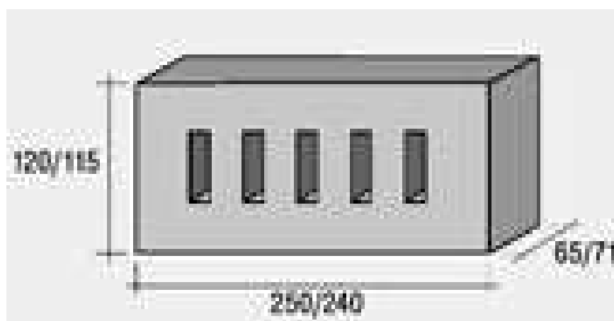
Ryc. 2 Cegła 5-szczelinowa
