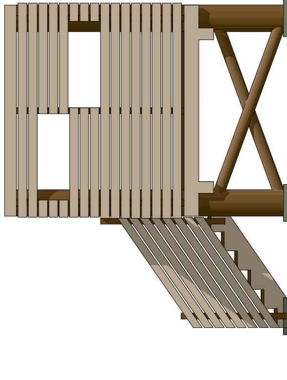
ELEWACJA PÓŁNOCNO-ZACHODNIA
