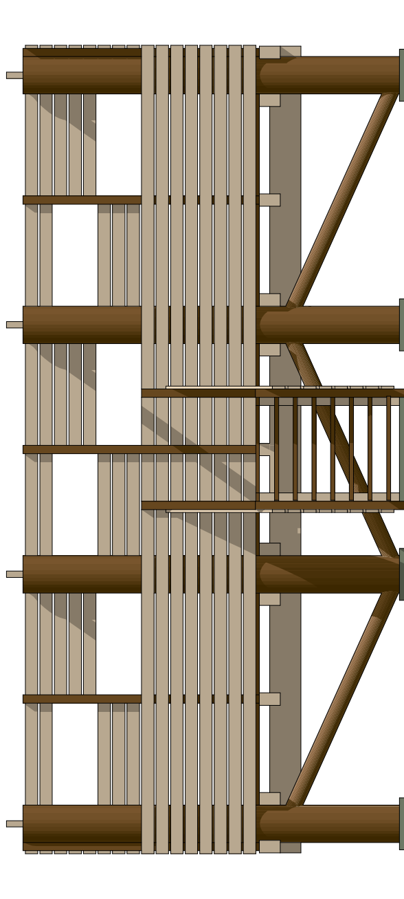
ELEWACJA POŁUDNIOWO-WSCHODNIA
